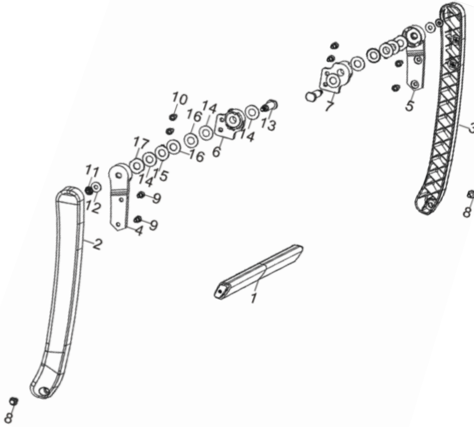
Fig. 15 - Handle
